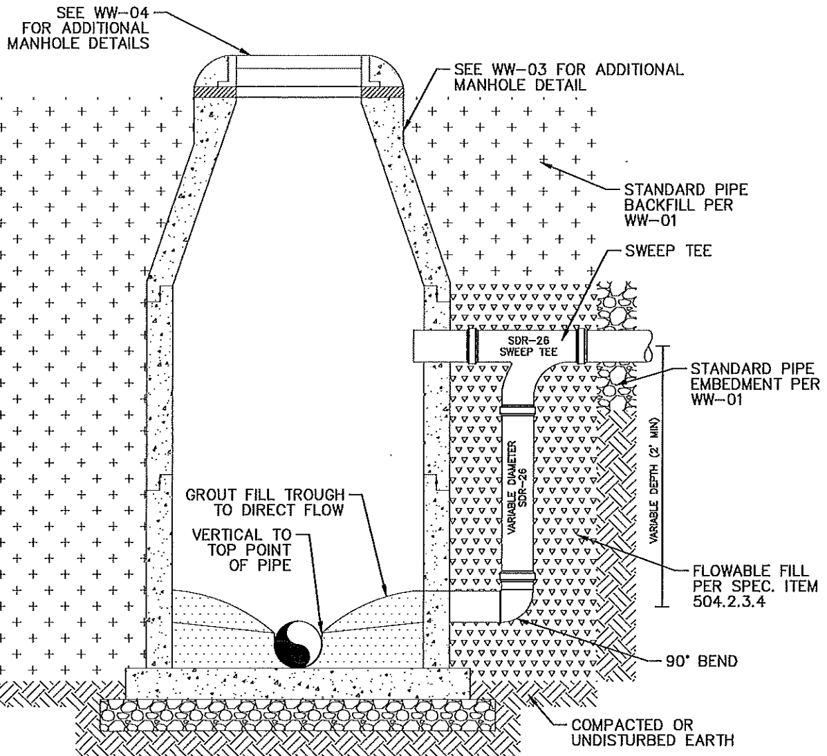
ELEVATION A
